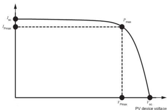
图1 光伏组件的电流-电压 ( I-V ) 特性曲线
